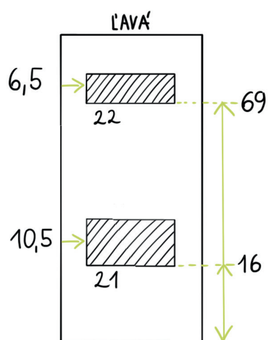
VÝREZY OKNA
